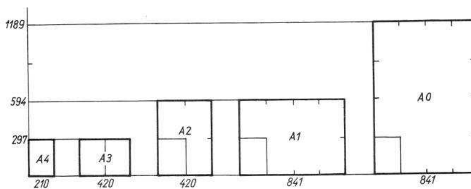
Związki między różnymi formatami rysunkowymi
